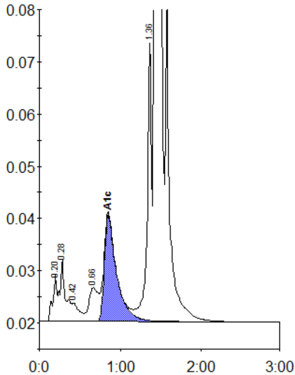
Peak table - ID: 10379976
